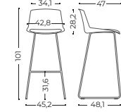
Cantilever stool Taburete Patín de acero
